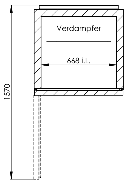
SCHNITT B-B
