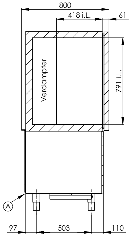
SCHNITT A-A
